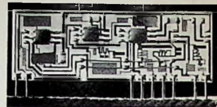
Spoelloze filters van Siemens in tantalium-dunnefilmtechniek, tesamen met een monolithisch geïntegreerde operationele schakelingen in één platte omhulling
